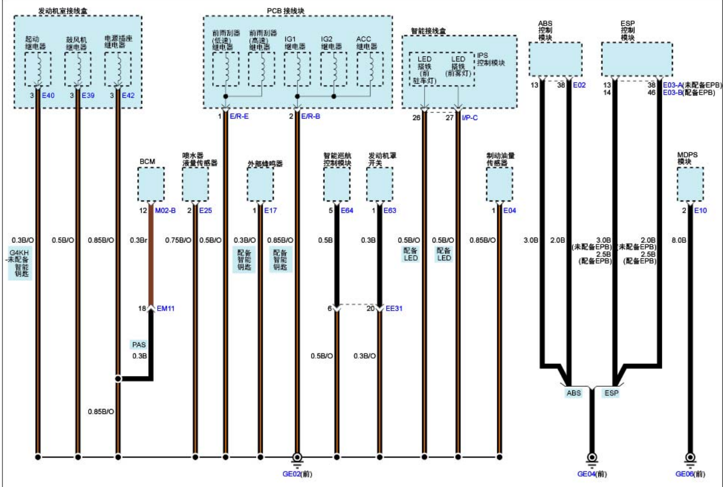
搭铁分布(6)
